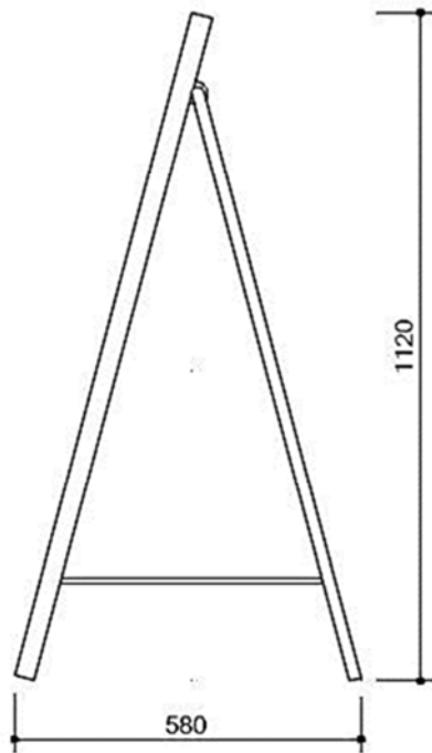
側面(設置時)
